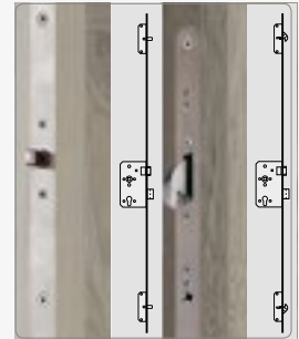
Dreifachverriegelung mit Rundbolzen oder Schwenkhaken
